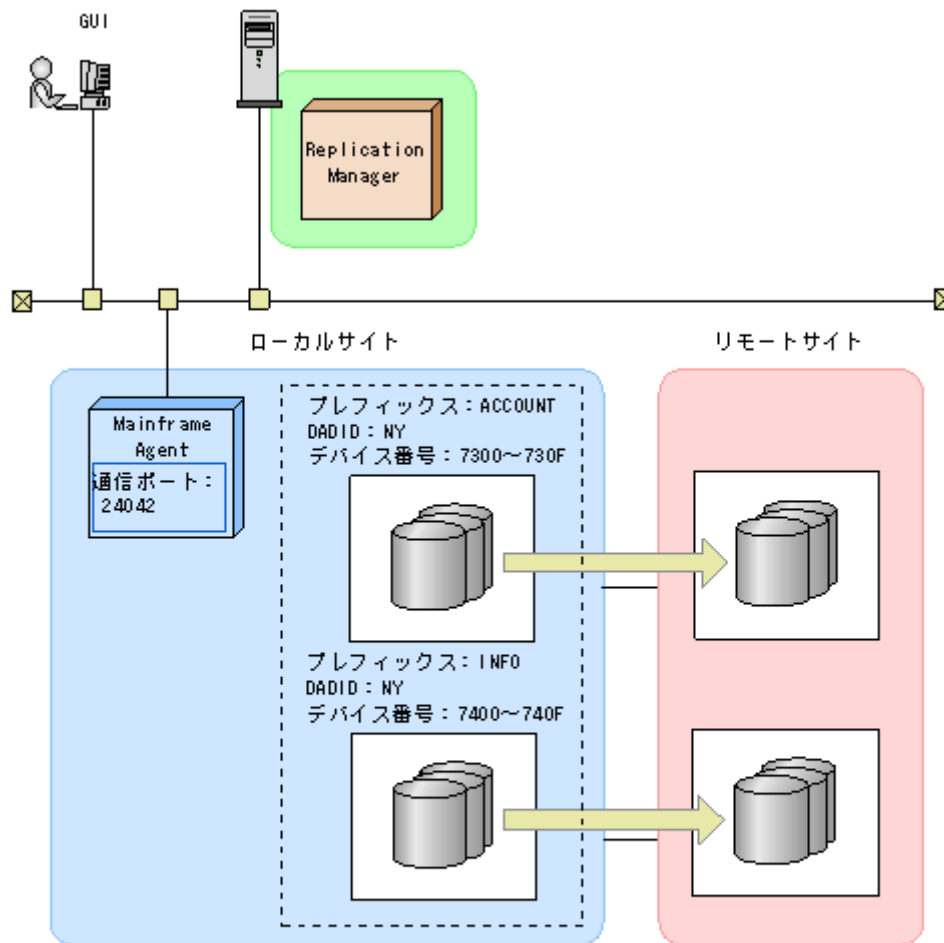
図 3-3 Replication Manager と接続する場合の構成例
