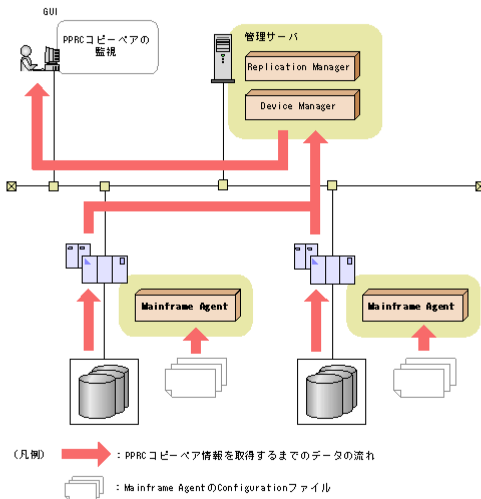
図 1-2 Replication Manager で PPRC コピーペアを監視するための構成
